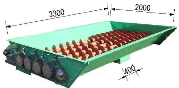
実際はスクリーの上に 1500φのトンネルがあります
